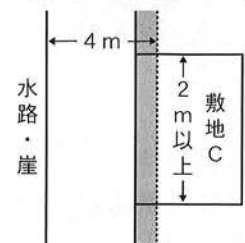
道路幅員が4 m未満の場合で片側が水路や崖などの場合
