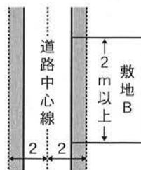
道路幅員が4 m未満の場合
